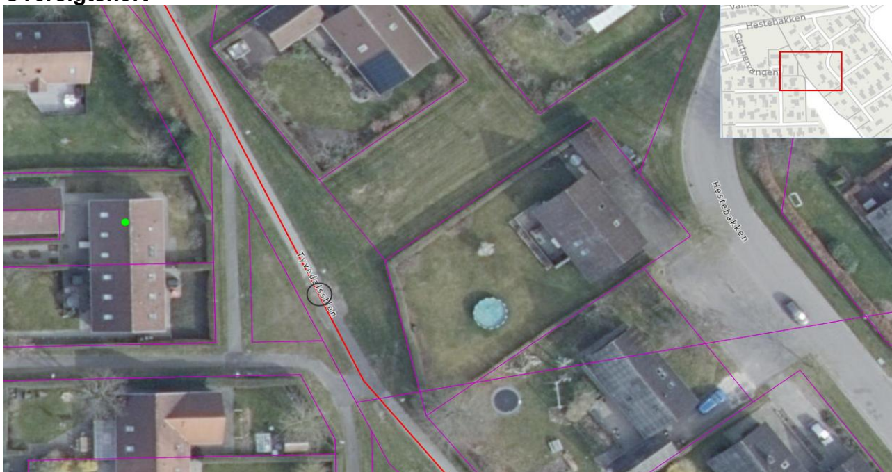
Figur 1 Oversigtskort over projektområdet. Den røde linje indikerer det rørlagte vandløb og den sorte cirkel markerer hvor krydsningen med spildevandsledningen foretages.
