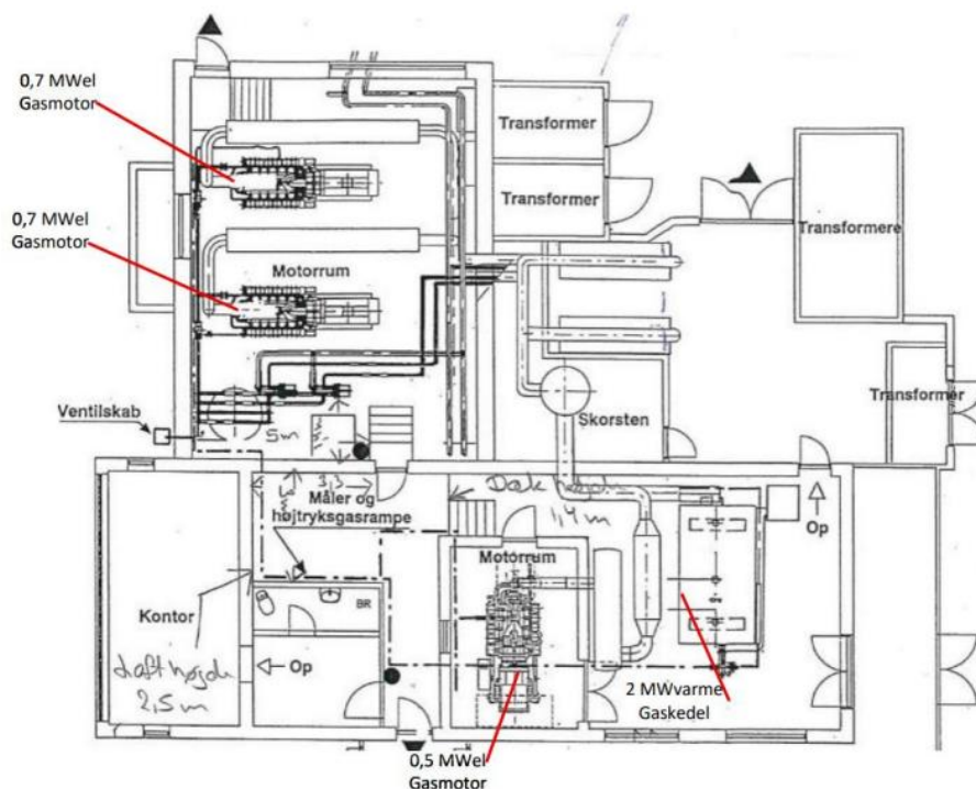
Figur 1: Nuværende situationsplan, Fælledvej 2
