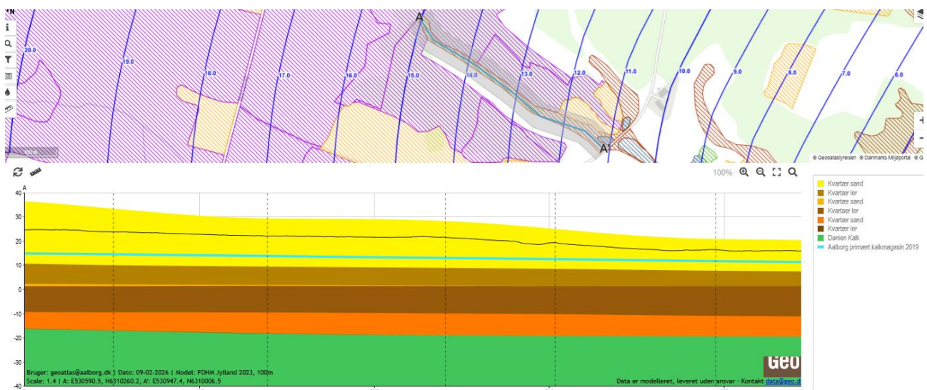
Figur 3. Tværsnit gennem naturlokalitet område 2, se figur 6 afsnit 4.2.3.1 'Hydrologisk vurdering af natur'. Kilde: FOHM (Fælles Offentlige Hydrostratigrafiske Model) og Aalborg Kommunes potentialekort 2019, tegnet i GeoAtlas.
