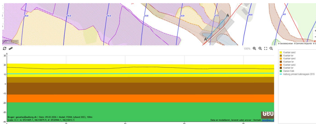
Figur 4. Tværsnit gennem naturlokalitet område 3 og 4, se figur 6 afsnit 4.2.3.1 'Hydrologisk vurdering af natur'. Kilde: FOHM (Fælles Offentlige Hydrostratigrafiske Model) og Aalborg Kommunes potentialekort 2019, tegnet i GeoAtlas.
