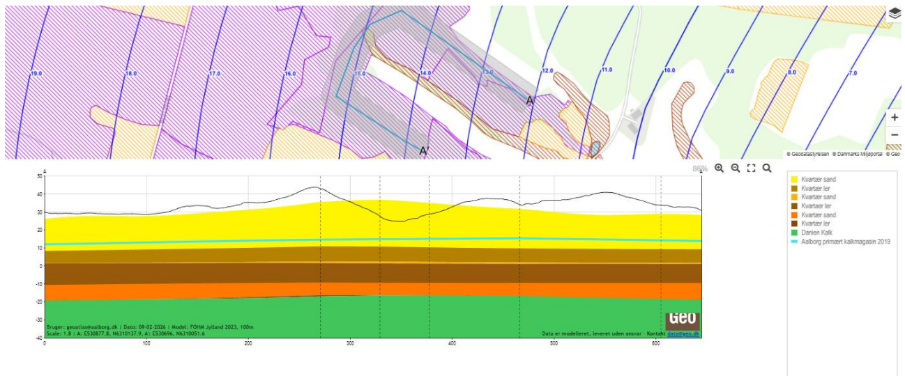
Figur 2. Tværsnit gennem naturlokalitet område 1, se figur 6 afsnit 4.2.3.1 'Hydrologisk vurdering af natur'. Kilde: FOHM (Fælles Offentlige Hydrostratigrafiske Model) og Aalborg Kommunes potentialekort 2019, tegnet i GeoAtlas.
