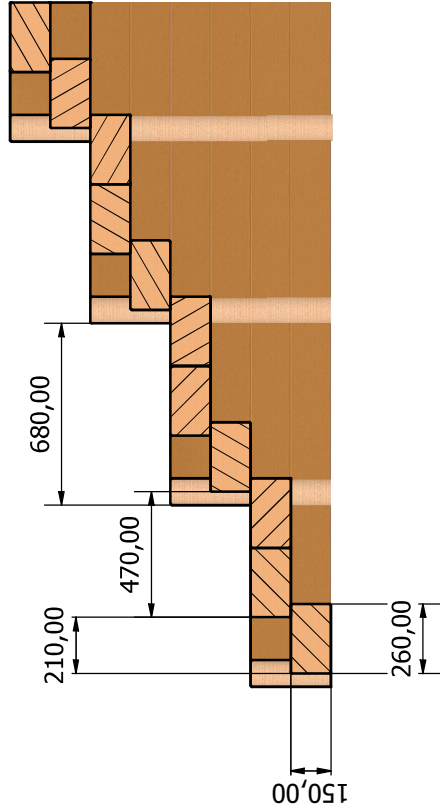
A-A ( 1:20 )
